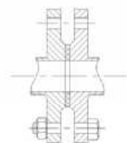
普通法兰-PN10kg
