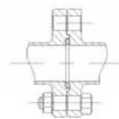
无菌法兰(可选) DIN11864-2-A
