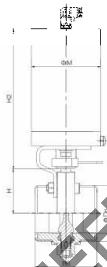
不锈钢气动蝶阀 SS Pneumatic butterfly valve NO.DS-VDF130Q1
