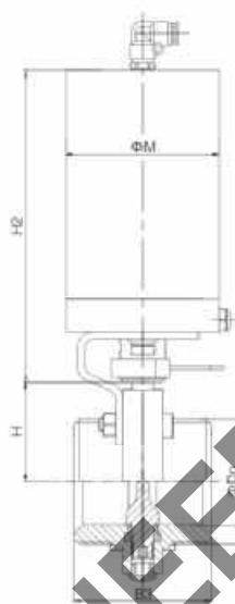
不锈钢气动蝶阀 SS Pneumatic butterfly valve NO.3A-VDF130Q1
