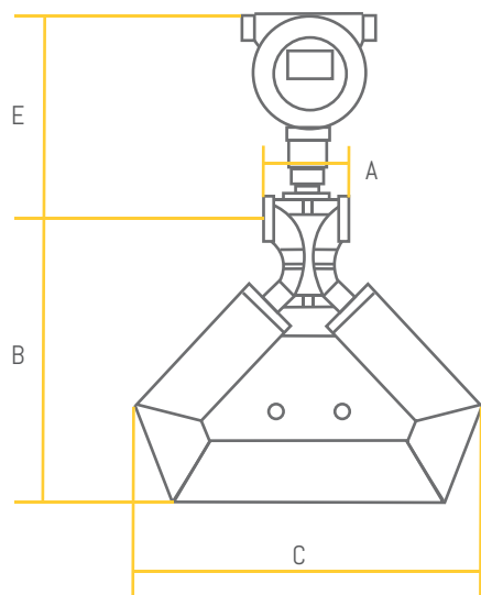
CMF 010/ 015 Compact Type
